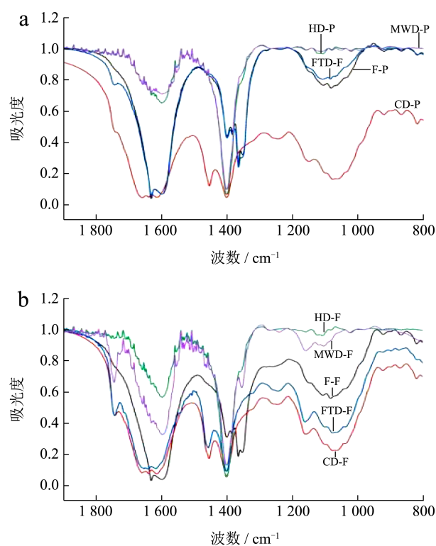
图9 不同脱水联合烹饪处理黄瓜钱儿纤维素傅里叶红外光谱图
