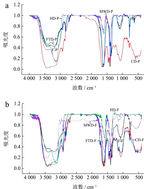
图 12 不同失水处理下黄瓜钱儿果胶傅里叶红外光谱图
