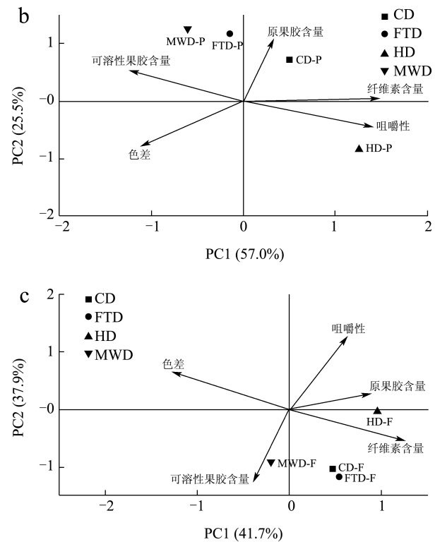
图 14 PCA 载荷图
