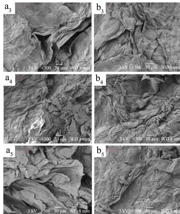
图 10 不同脱水联合烹饪处理黄瓜钱儿纤维素扫描电子显微镜图片
