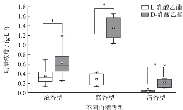
图 6 不同香型白酒中 D-乳酸乙酯和 L-乳酸乙酯的含量箱线图
