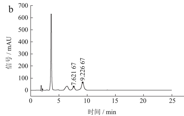
图 1 乳酸对映体色谱图
