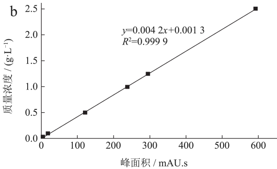
图 3 乳酸对映体标准曲线
