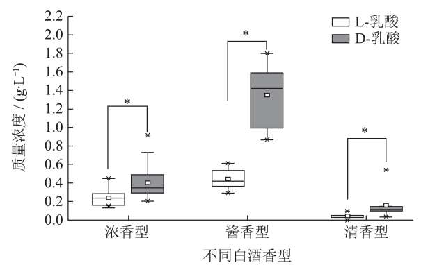
图 5 不同香型白酒中 L-乳酸和 D-乳酸的含量箱线图 Fig.5 Box plot of L-lactic acid and D-lactic acid content in different flavor liquors
