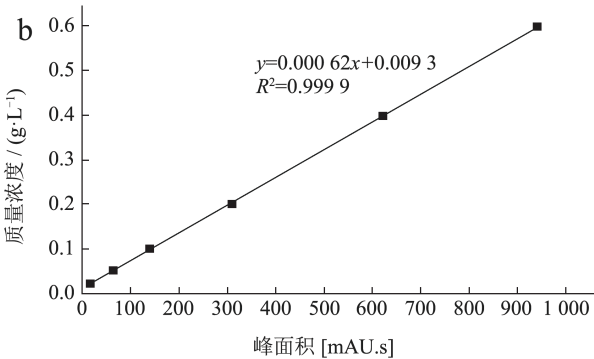
图 4 乳酸乙酯对映体的标准曲线
