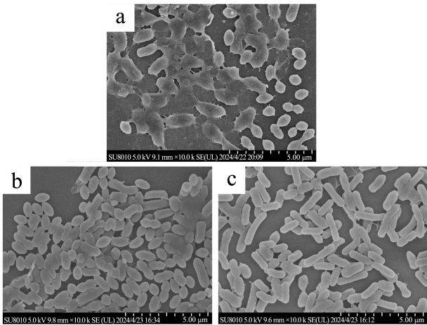
图 4 扫描电镜下不锈钢表面、玻璃表面和塑料表面 P. fluorescens 18 形成的生物膜形态
