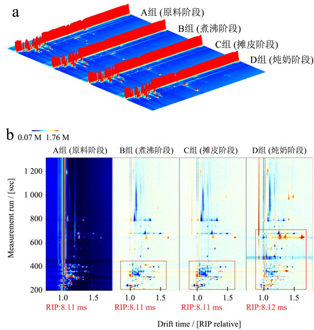
图3 HS-GC-IMS 检测挥发性物质结果 Fig.3 Results of volatile compound detection by HS-GC-IMS 注：(a) 3D 地形图：信号峰横坐标表示挥发性物质的迁移时间，纵坐标表示保留时间，信号峰体积表示其挥发性物质的浓度。(b) 二维差异报告图：反应离子峰（Reactive Ion Peak, RIP）两侧的颜色斑点是物质的响应信号峰，其颜色深浅显示物质浓度。以 A 组为对照，蓝色斑点指风味化合物含量低于 A 组数值，红色斑点则表示高于 A 组数值。
