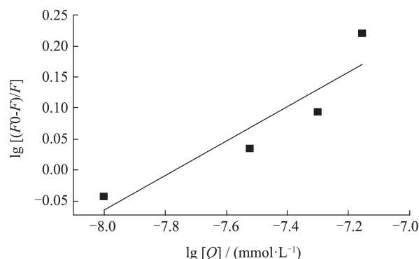
图 6 298 K 下香菇多酚对 \alpha -葡萄糖苷酶相互作用的双对数曲线
