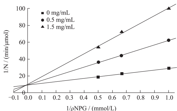
图3 香菇多酚对 \alpha -葡萄糖苷酶抑制作用的 Lineweaver-Burk 图
