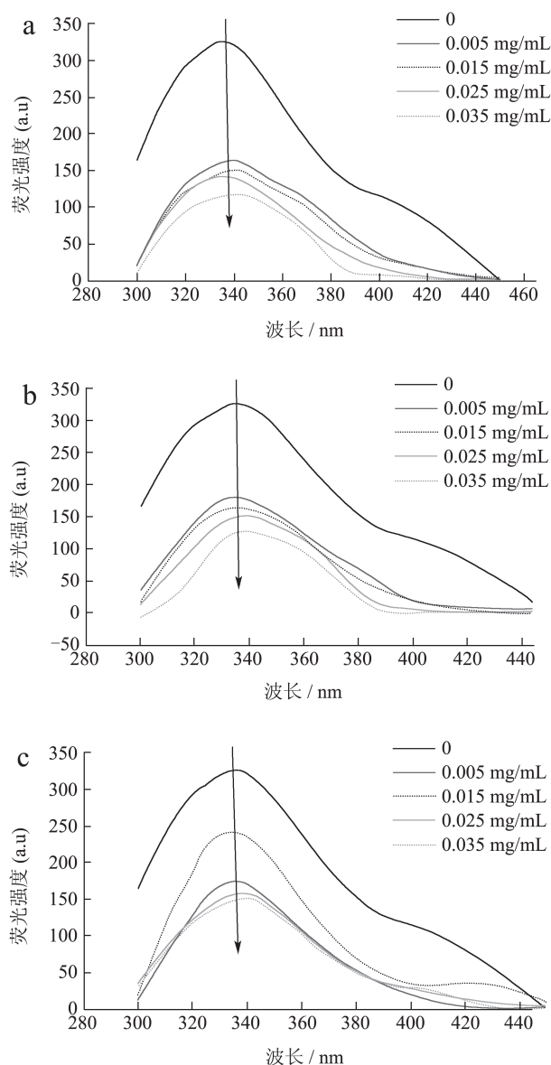
图4 不同温度下香菇多酚对 \alpha -葡萄糖苷酶荧光光谱的影响
