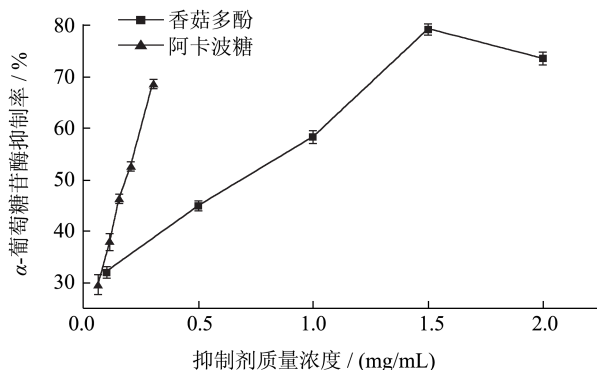
图1 香菇多酚与阿卡波糖对 \alpha -葡萄糖苷酶的抑制作用
