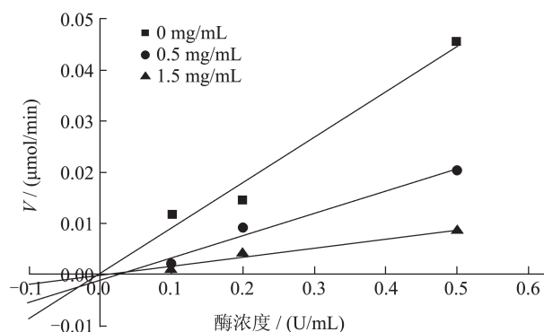
图2 香菇多酚对 \alpha -葡萄糖苷酶活性的抑制动力学曲线
