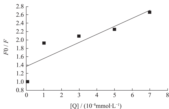
图 5 298 K 下香菇多酚与 \alpha -葡萄糖苷酶相互作用的 Stern-Volmer 方程曲线图
