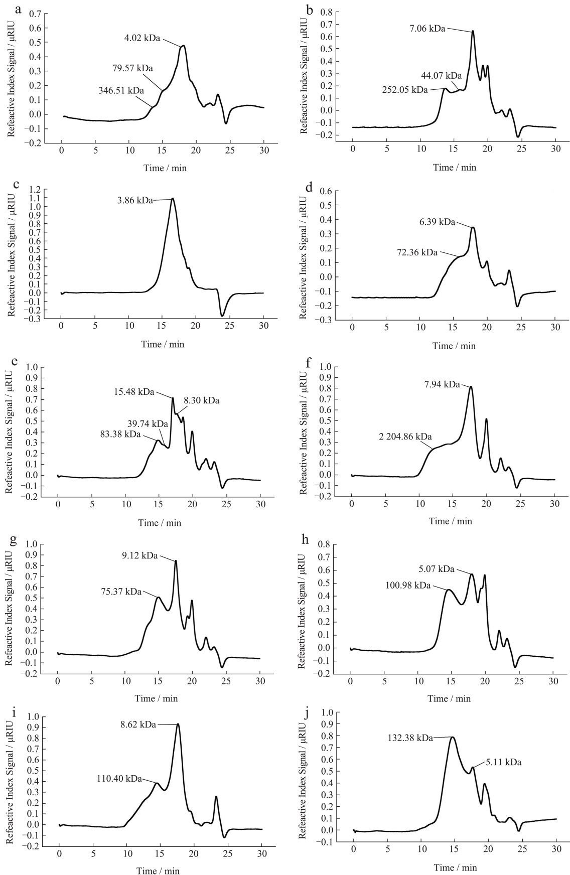
图 1 10 款蓝莓酒中多糖分子量分布图
