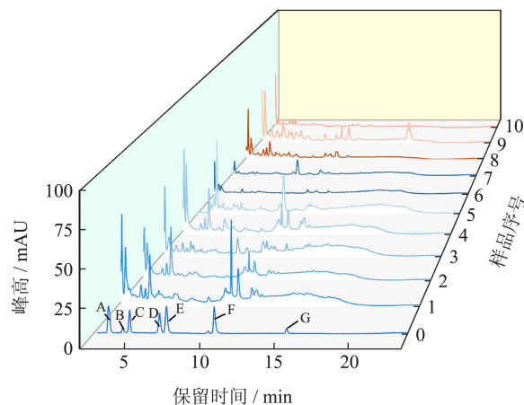
图3 10款蓝莓酒维生素色谱图
