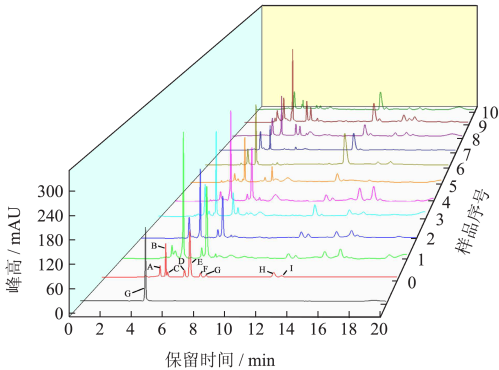
图 2 10 款蓝莓酒有机酸色谱图
