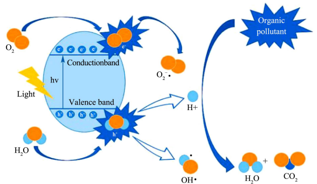
图 4 光催化降解机理
