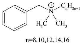
图 1 苯扎氯铵化学结构
