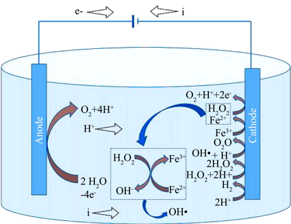
图 6 Fenton 氧化工艺
