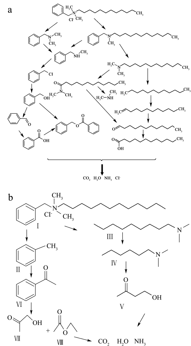
图 7 Fenton 氧化降解 BACs 机制
