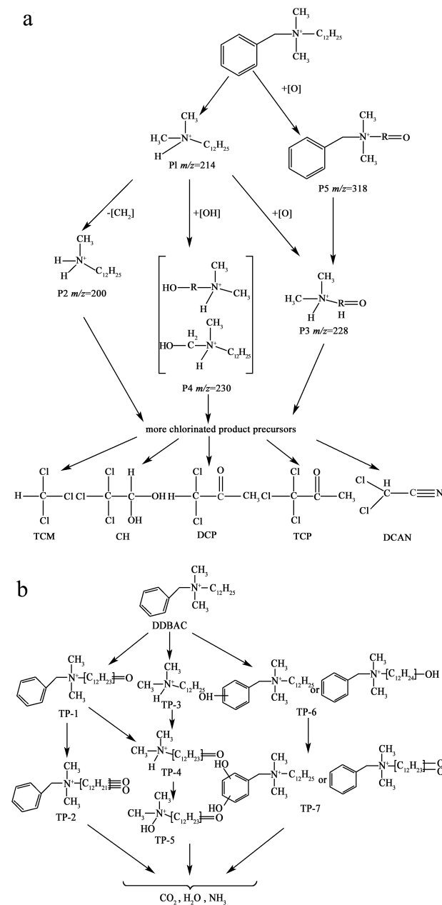
图 5 光催化降解 DDBAC 的途径
