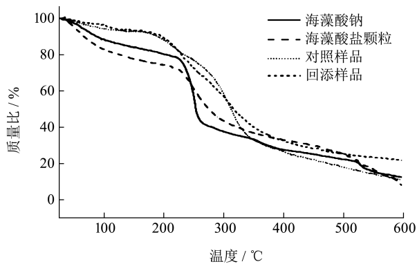
图 3 不同样品的热重分析曲线
