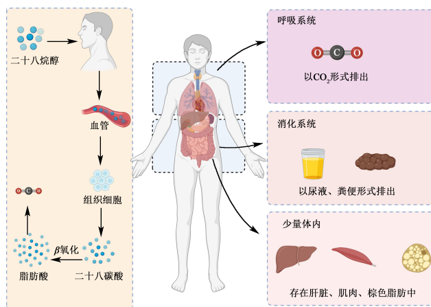
图4 二十八烷醇吸收代谢
