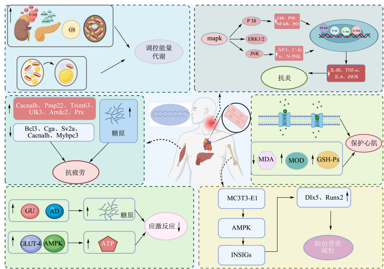
图 3 二十八烷醇药理机制 Fig.3 Pharmacological mechanisms of octacosanol
