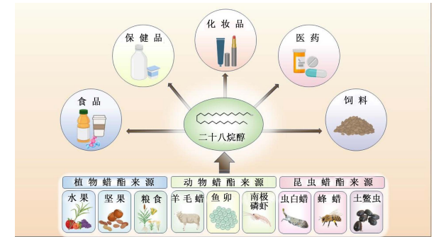
图 1 二十八烷醇的来源及应用 Fig.1 Sources and applications of octacosanol
